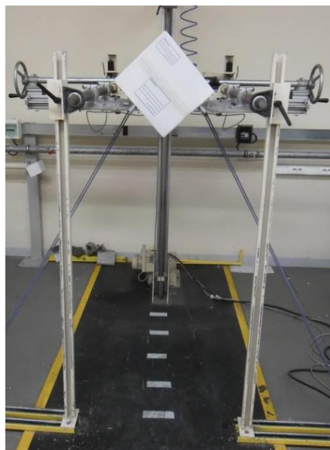
Figura 4 Esempio di caduta su uno spigolo
