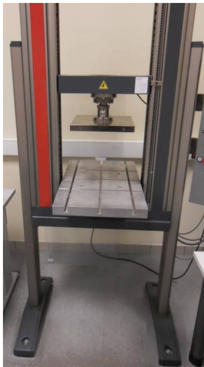
Figura 2 Macchina di trazione-compressione Zwick
